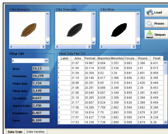
Gambar 4 Screenshot simulasi proses ekstraksi fitur
