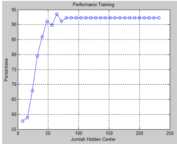
Gambar 5 Performa pelatihan
