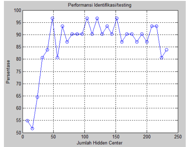
Gambar 6 Performa pengujian
